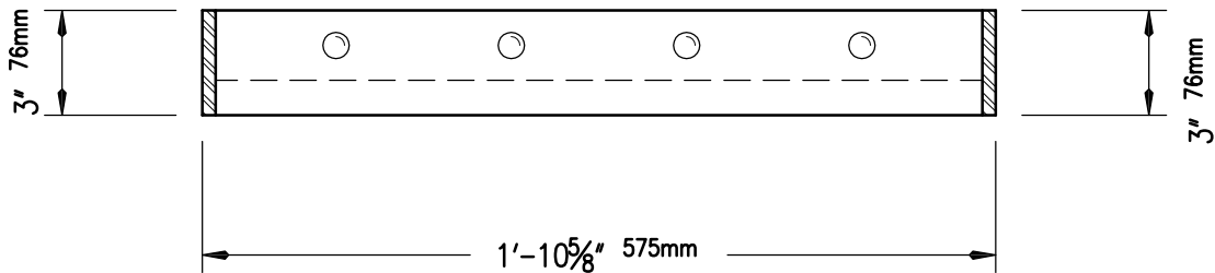
SIDE ELEVATION SCALE: 2"=1'-0"
